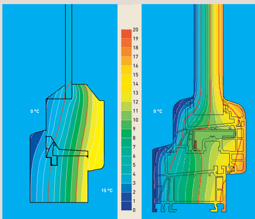
Ancienne fenêtre bois simple vitrage U_w moyen 5,8 \text{ W}/(\text{m}^2.\text{K})
