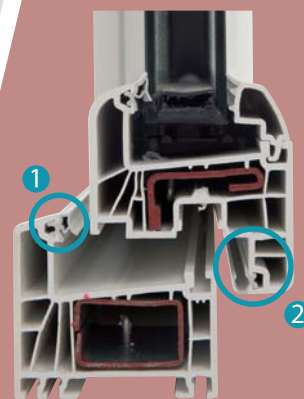
Système d'étanchéité à 2 joints
