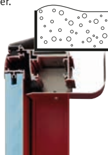
Vue de coupe coffre linteau.
