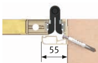
Pose entre tableaux
