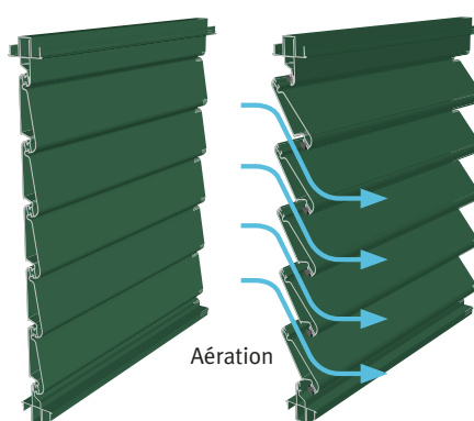
Coupe verticale Lames orientables
