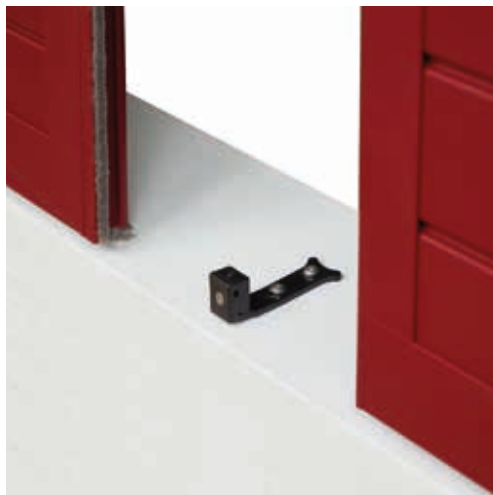
La dardenne sur appui de fenêtre permet le blocage des volets en position fermée.
