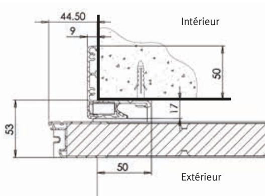
Coupe sur précadre
