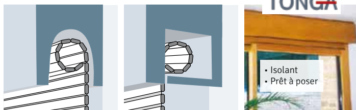
coffre linteau
